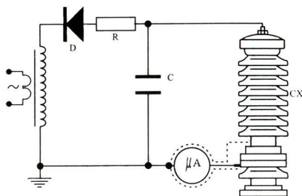
排除试品CX表面影响接线图
