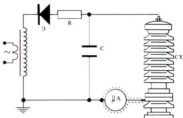
微安表接入试品CX底部的接线图
