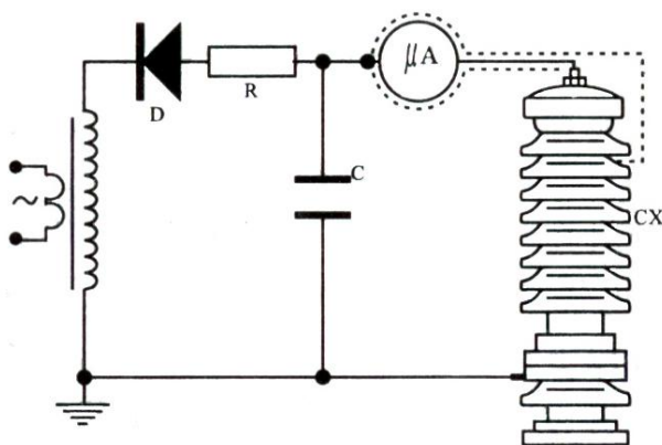
排除试品CX表面影响接线图
