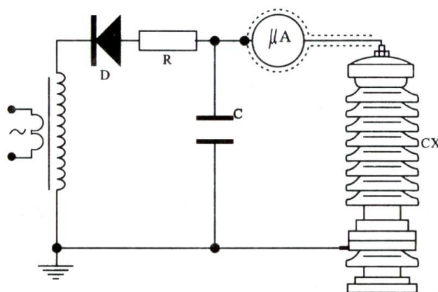
微安表接入试品CX高压侧接线图
