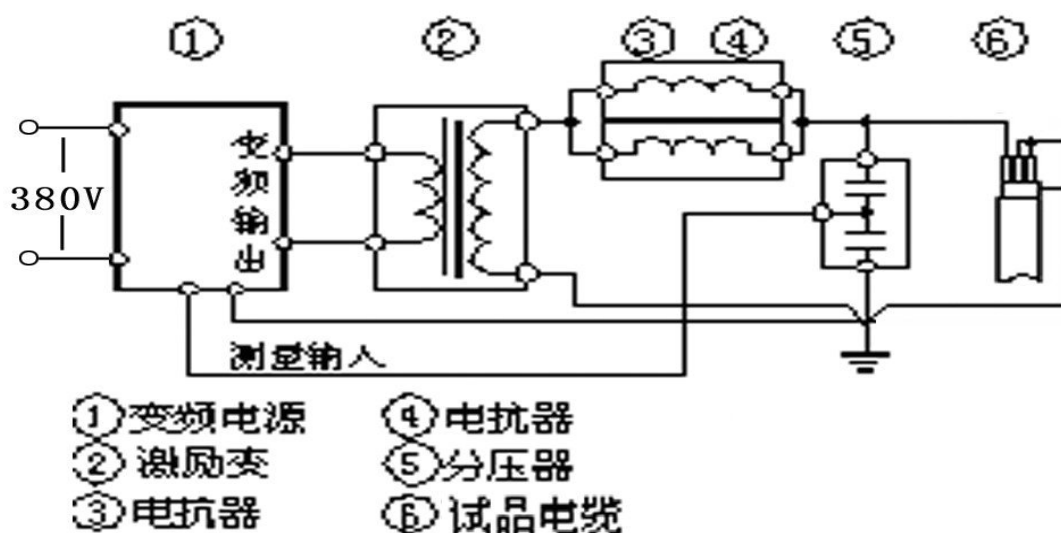
电缆耐压试验接线图
