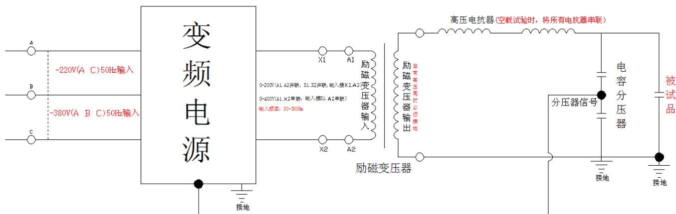
调频谐振试验接线示意图
